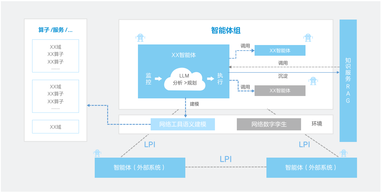
图04 多智能体群智协同
